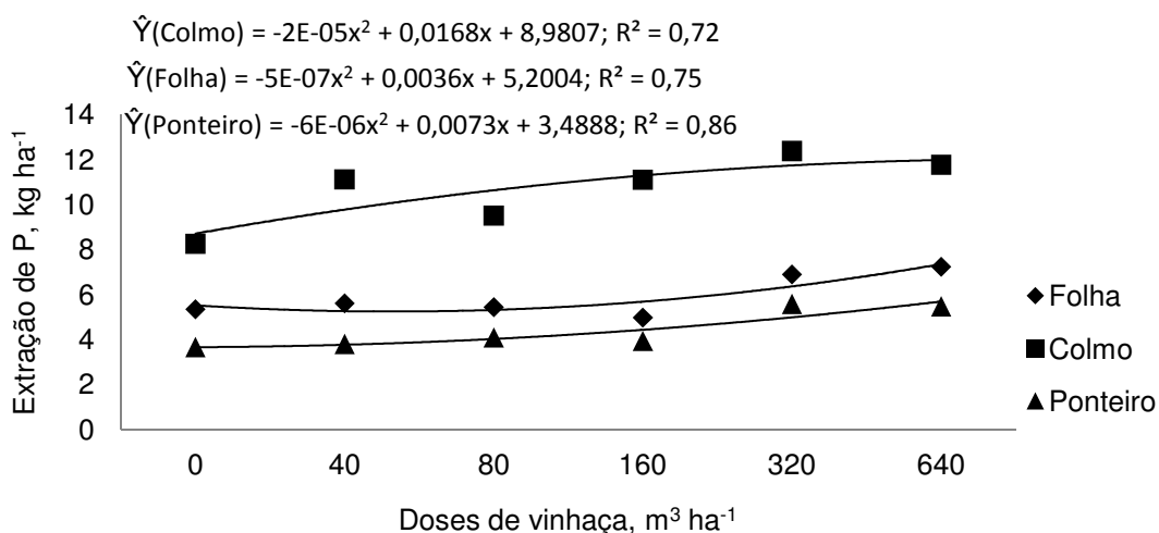
Figura 24. Extração de fósforo (P) em folhas, colmo e ponteiro de cana-de-açúcar, cultivar RB92579, em função das doses de vinhaça 0, 40, 80, 160, 320 e 640 m 3 ha -1 aos 240 DAP.
